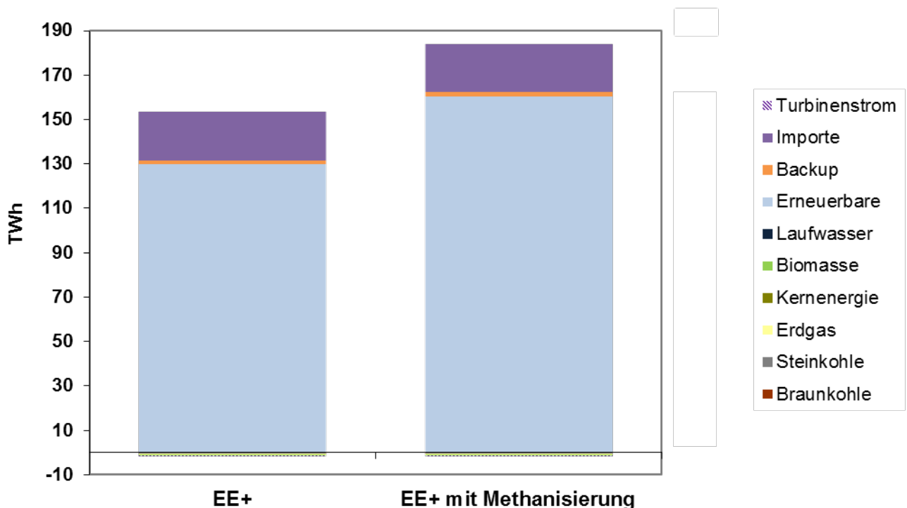
Abbildung 5-17: Vergleich Differenzstrom ohne und mit Sensitivität Methanisierung EE-Überschuss ( Grenzenlos eMobil 2050 )
