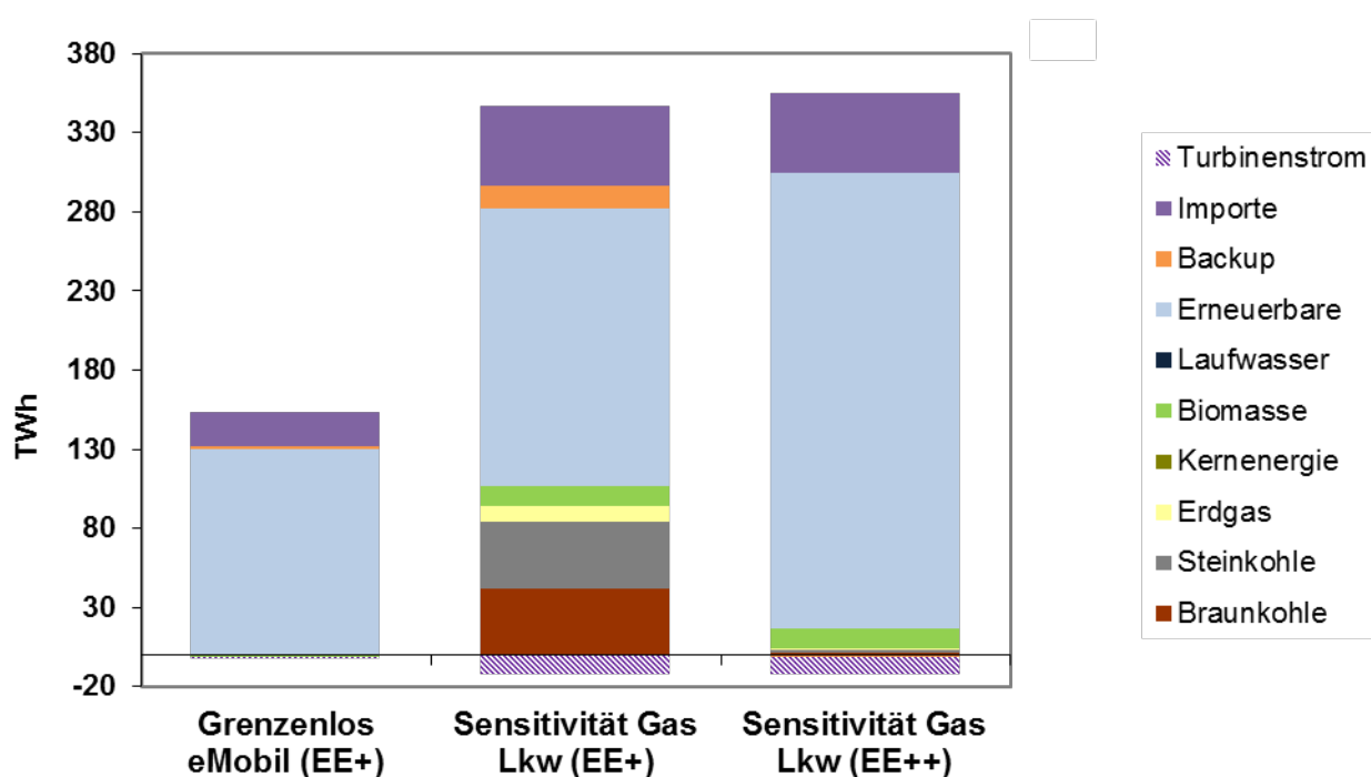
Abbildung 5-20: Vergleich Differenzstrom für die Sensitivität Gas-Lkw und PtG für Grenzenlos eMobil 2050
