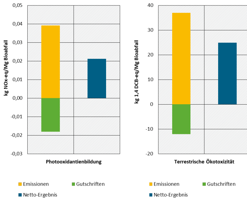
Abbildung 31: Ökobilanzergebnisse (Wirkungskategorien Photooxidantienbildung, terrestrische Ökotoxizität) für die hydrothermale Carbonisierung
