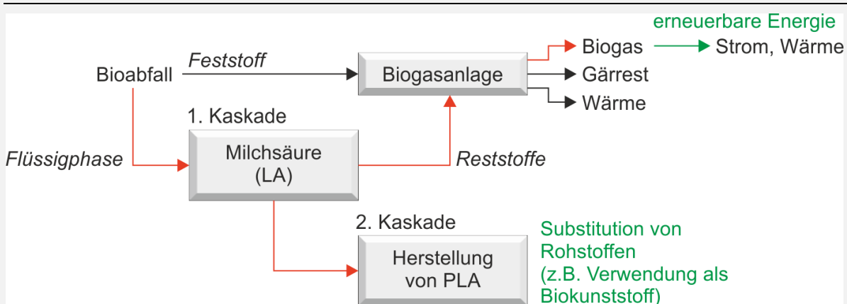
Abbildung 21: Schematische Darstellung einer um eine Milchsäurefermentation erweiterte Vergärungsanlage
