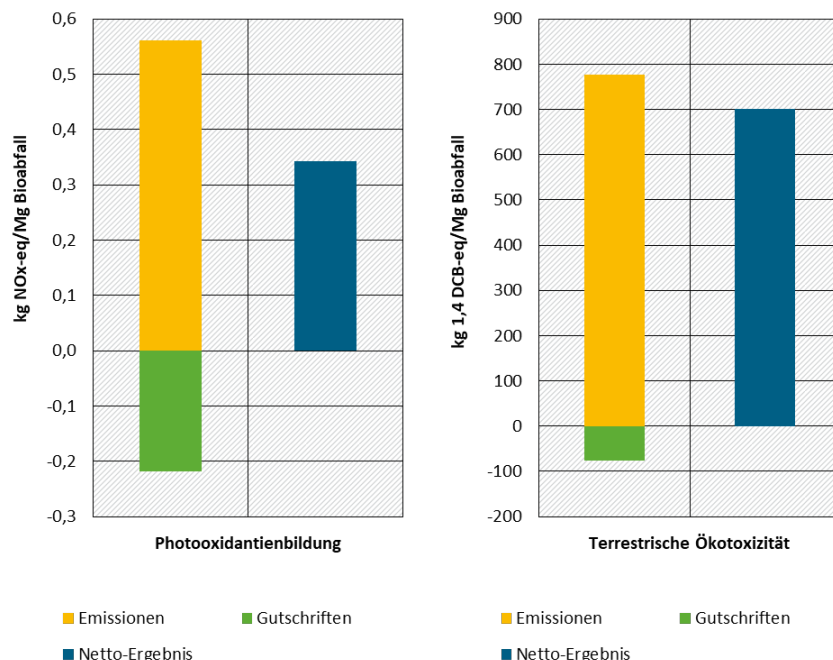
Abbildung 37: Ökobilanzergebnisse (Wirkungskategorien Photooxidantienbildung, terrestrische Ökotoxizität) für das HTV-Verfahren
