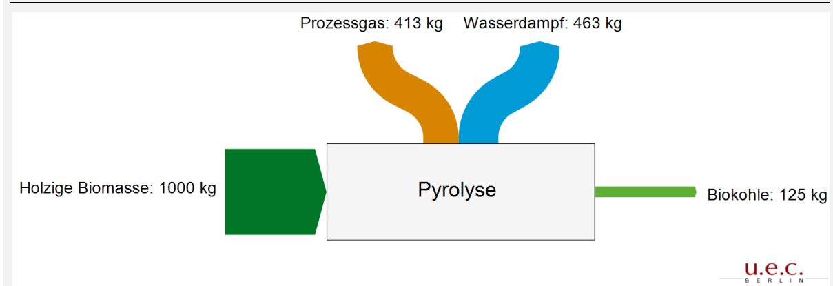
Abbildung 9: Vereinfachte Massenbilanz einer Pyrolyse-Anlage, WG des Inputmaterials < 50 %
