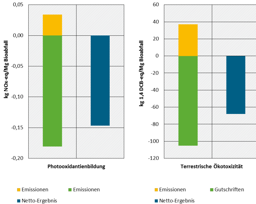
Abbildung 34: Ökobilanzergebnisse (Wirkungskategorien Photooxidantienbildung, terrestrische Ökotoxizität) für die Pyrolyse
