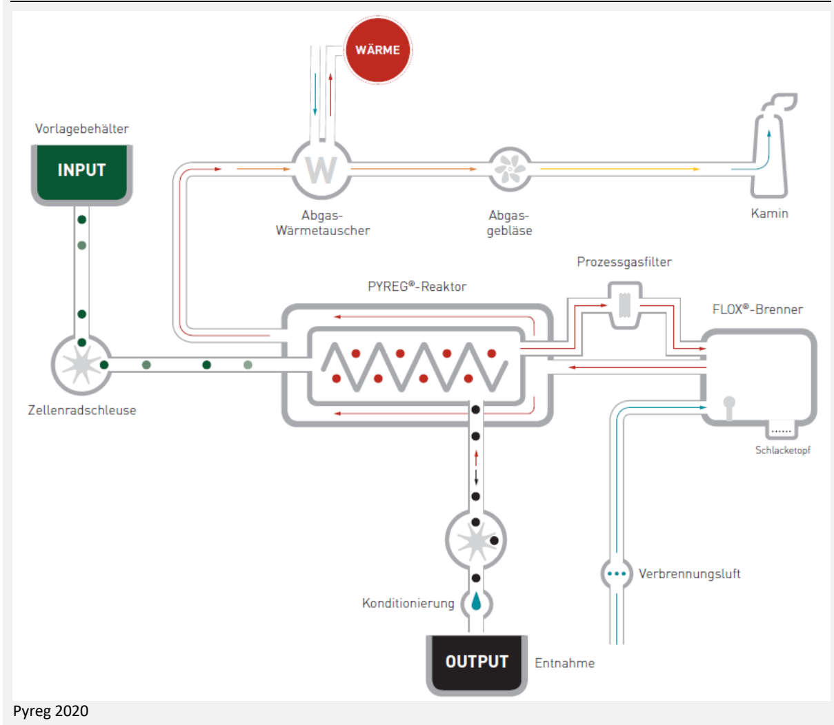
Abbildung 8: Vereinfachtes Prozessschema des Pyreg®-Verfahrens
