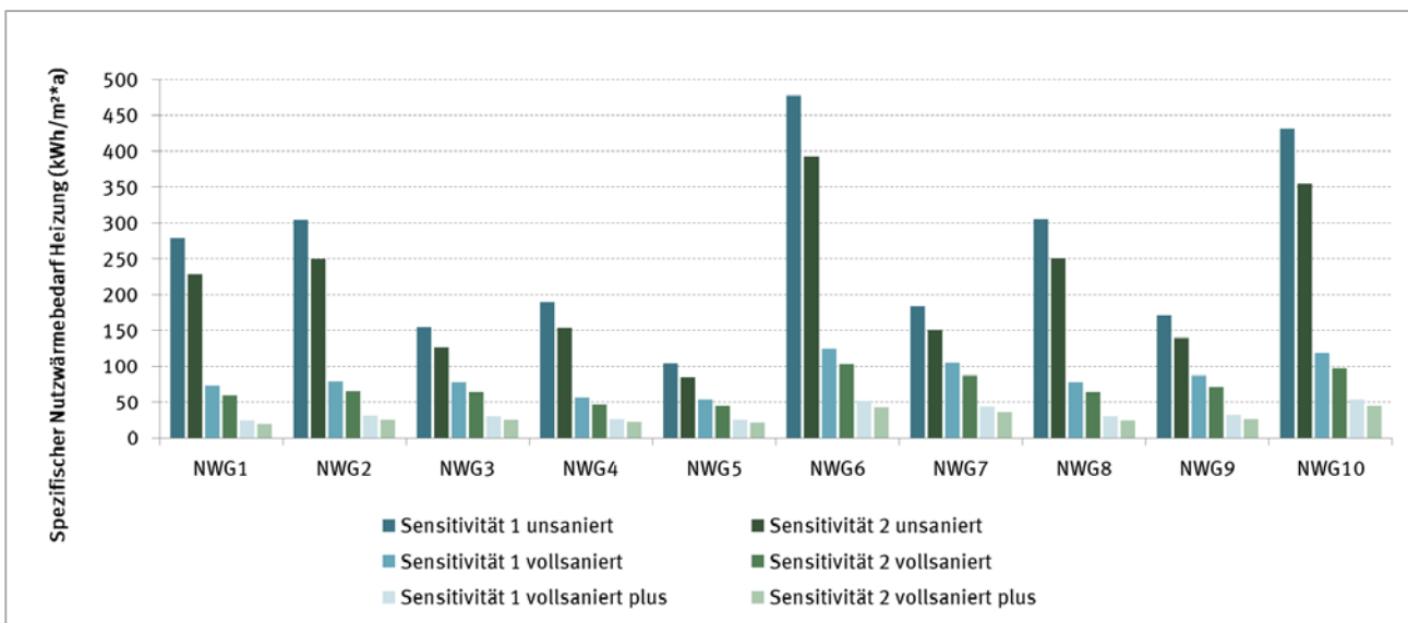
Abbildung 63: Spezifischer Nutzenergiebedarf für Heizung aufgrund der erwarteten Klimaveränderungen (Referenzstandort Potsdam)
