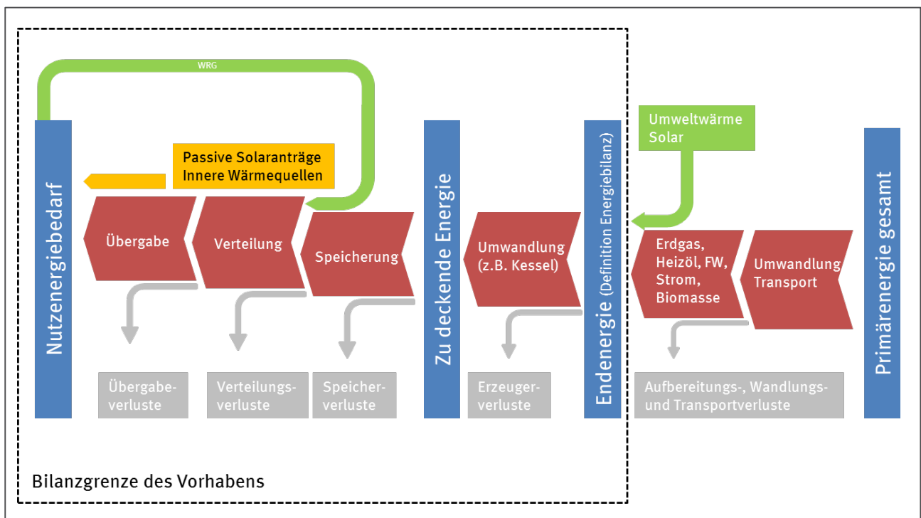
Abbildung I: Schematisches Energieflussbild
