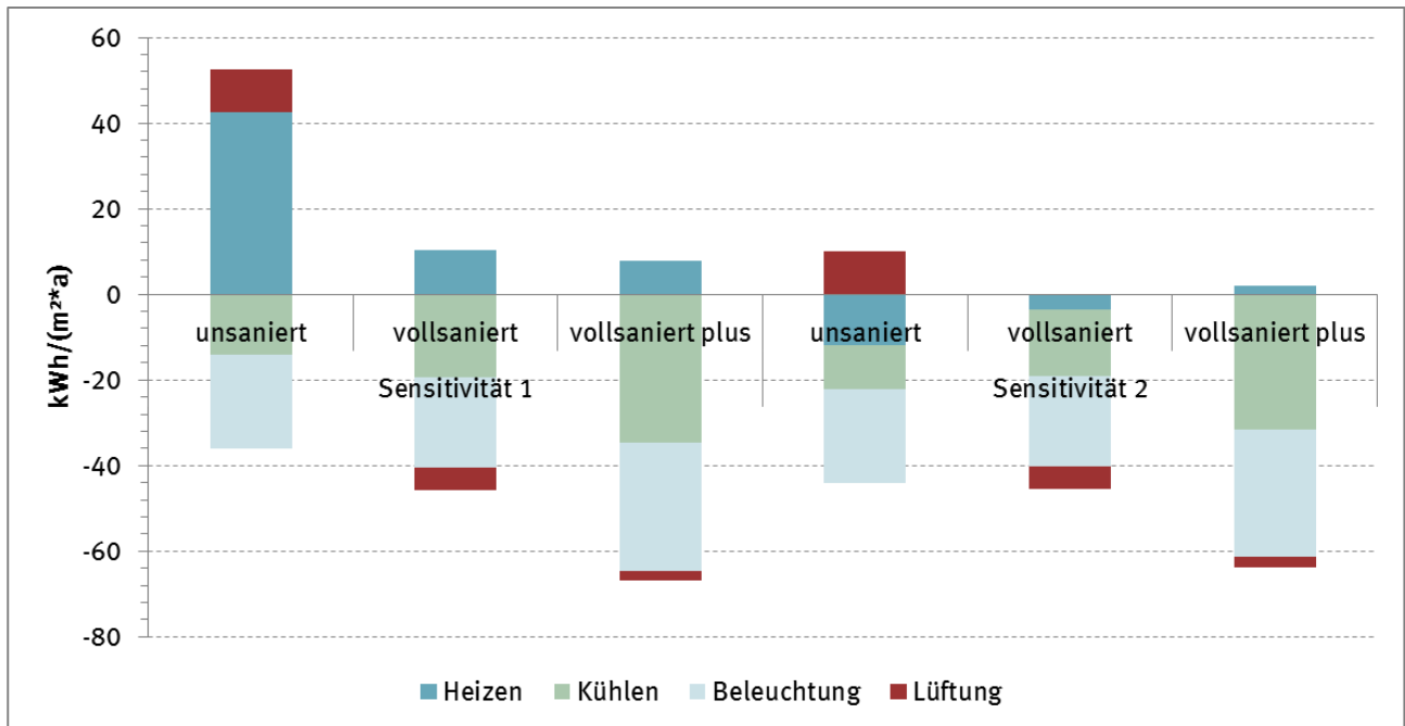
Abbildung 65: Exemplarische Darstellung der Veränderung des spezifischen Endenergieverbrauchs des NWG2 (Wärmebereitstellung durch Gas-Brennwertkessel, Kälteübergabe über TABS) der Sensitivitäten 1 und 2 gegenüber der Basis
