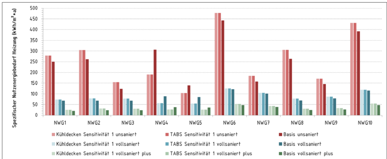
Abbildung 53: Spezifischer Nutzenergiebedarf für die Heizung der betrachteten Nichtwohngebäude und Sanierungsstandards, jeweils im Vergleich zur Basisvariante
