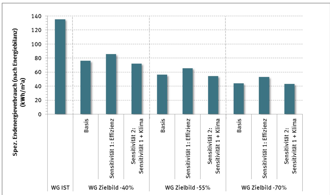
Abbildung 66: Durchschnittlicher spezifischer Endenergieverbrauch in den verschiedenen Zielbildern und Sensitivitäten der Wohngebäude
