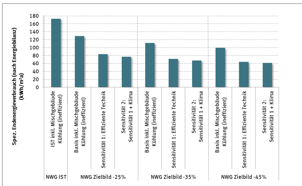
Abbildung 69: Durchschnittlicher spezifischer Endenergieverbrauch in den verschiedenen Zielbildern und Sensitivitäten der Nichtwohngebäude
