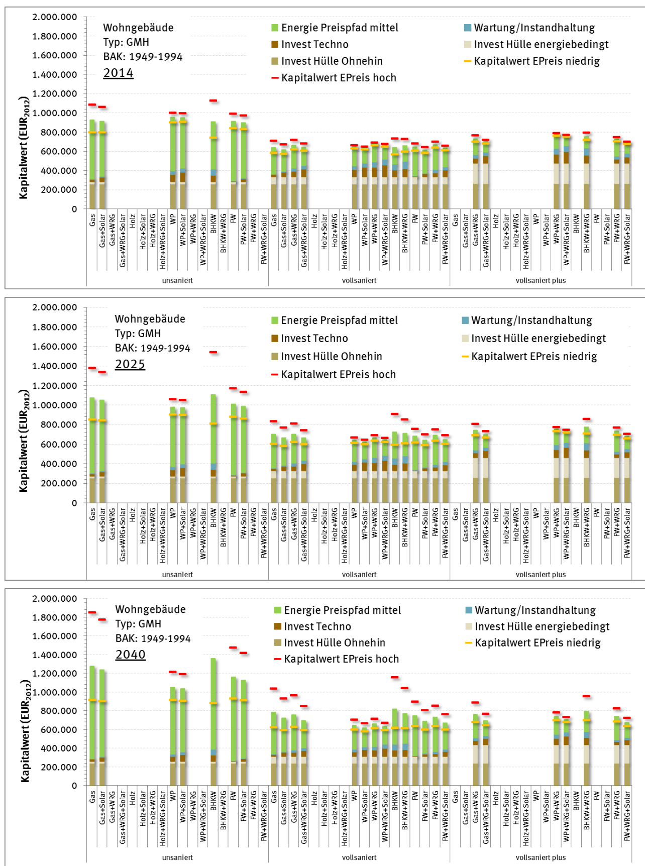
Abbildung 18: Kapitalwerte für ein GMH in Abh. von Versorgungstechnik, Wärmeschutzstandard und Investitionszeitpunkt
