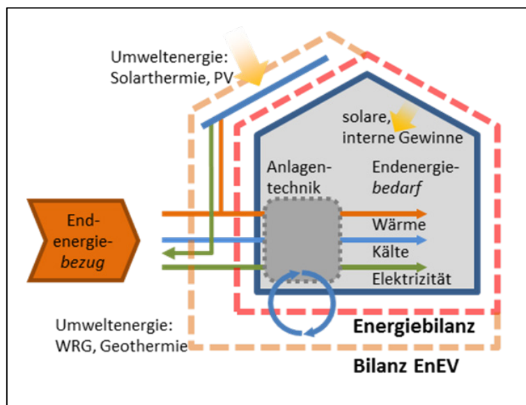
Abbildung 2: Bilanzgrenze Gebäude 9
