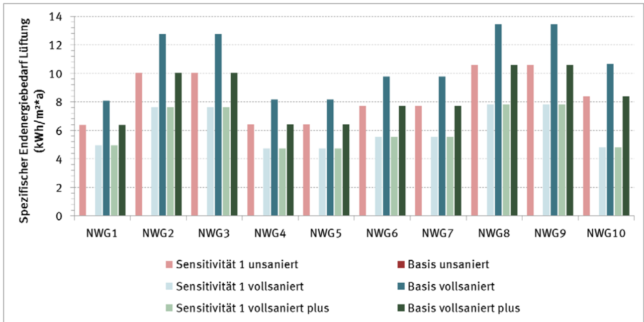
Abbildung 51: Spezifischer Endenergiebedarf für die Lüftung der betrachteten Nichtwohngebäude und Sanierungsstandards, jeweils im Vergleich zur Basisvariante
