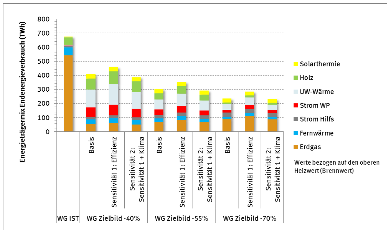
Abbildung 67: Energieträgermix des Endenergieverbrauchs (im Sinne der Energiebilanz) in den verschiedenen Zielbildern und Sensitivitäten der Wohngebäude
