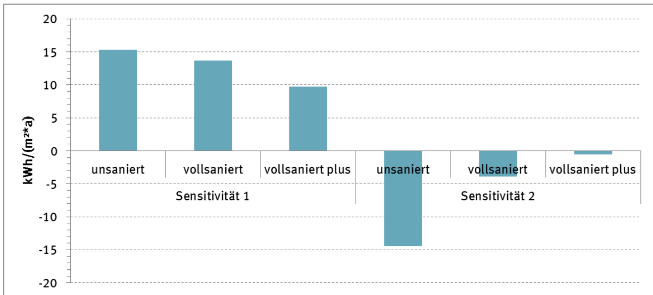
Abbildung 64: Exemplarische Darstellung der Veränderung des spezifischen Endenergieverbrauchs des EZFH mit BAK ab 1994 (Wärmebereitstellung durch Gas-Brennwertkessel) der Sensitivitäten 1 und 2 gegenüber der Basisvariante
