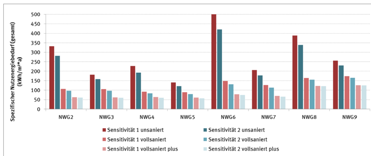
Abbildung 57: Spezifischer Nutzenergiebedarf (gesamt) in vorwiegend durch Kühldecken gekühlten Nichtwohngebäuden (NWG2-9) aufgrund der erwarteten Klimaveränderungen (Referenzstandort Potsdam)
