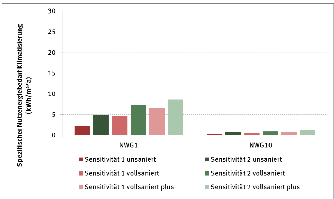
Abbildung 62: Spezifischer Nutzkältebedarf in vorwiegend durch Ventilator-konvektoren gekühlten Nichtwohngebäuden aufgrund der erwarteten Klimaveränderungen (Referenzstandort Potsdam)
