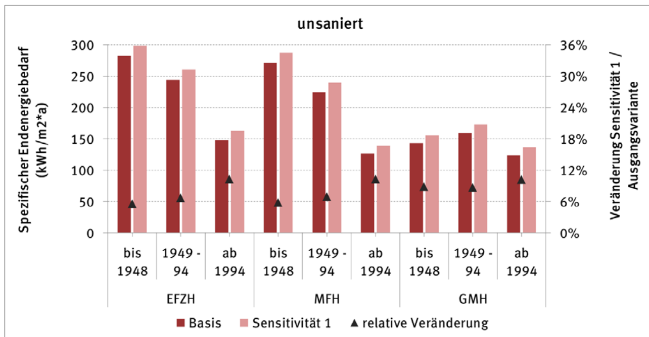
Abbildung 50: Spezifischer Endenergiebedarf für Heizung und TWW in Wohngebäuden (Gas-Brennwert) sowie die Veränderungen gegenüber der Basisvariante in Abhängigkeit vom Sanierungsstandard
