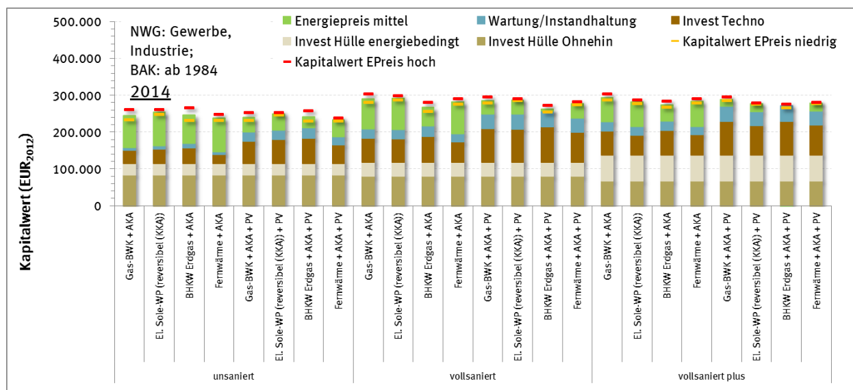
Abbildung 21: Kapitalwerte für Gewerbe- und Industriegebäude in Abh. von Versorgungstechnik, Wärmeschutzstandard und Investitionszeitpunkt
