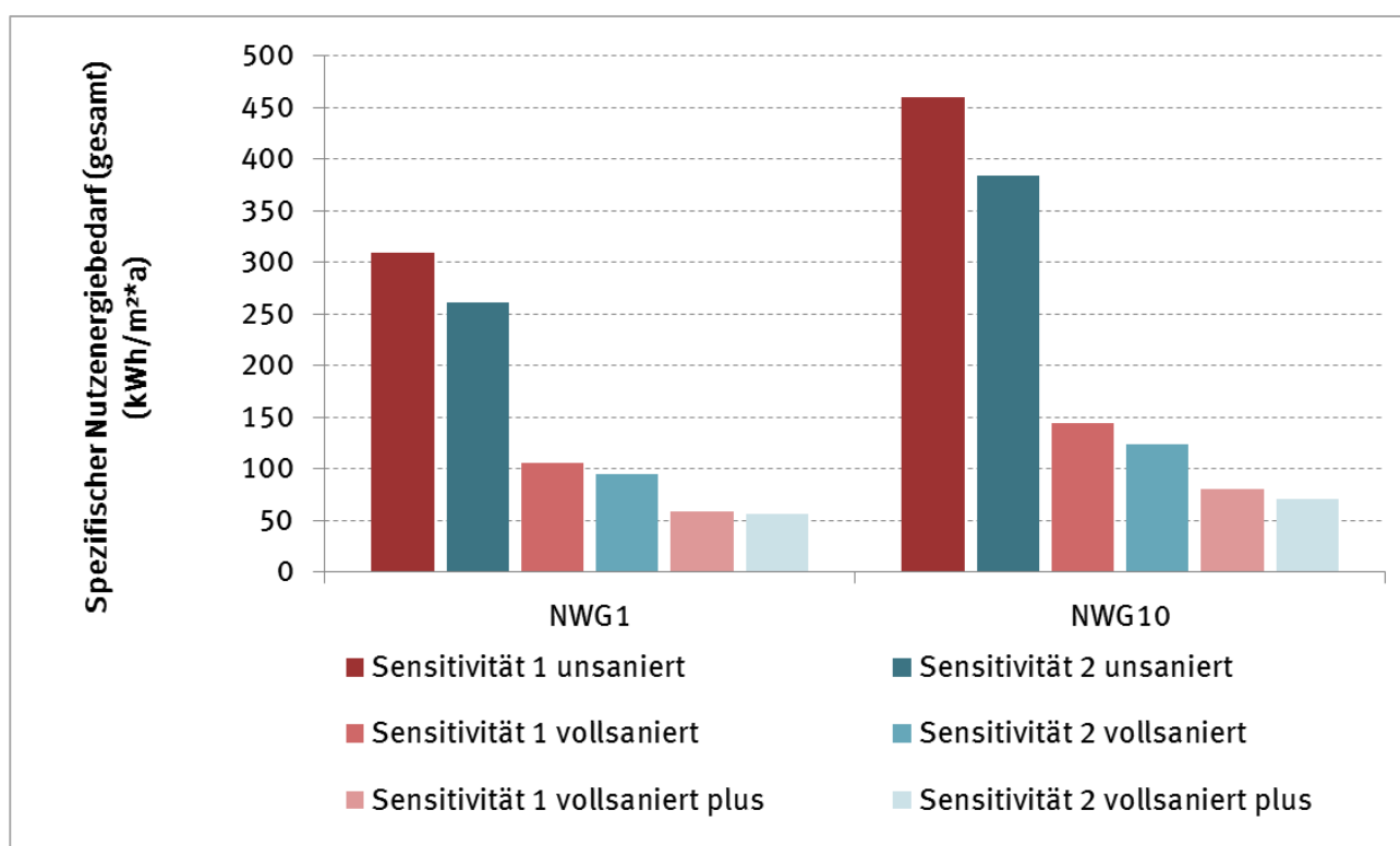
Abbildung 59: Spezifischer Nutzenergiebedarf (gesamt) in vorwiegend durch Ventilator-konvektoren gekühlten Nichtwohngebäuden (NWG1 und NWG10) aufgrund der erwarteten Klimaveränderungen (Referenzstandort Potsdam)
