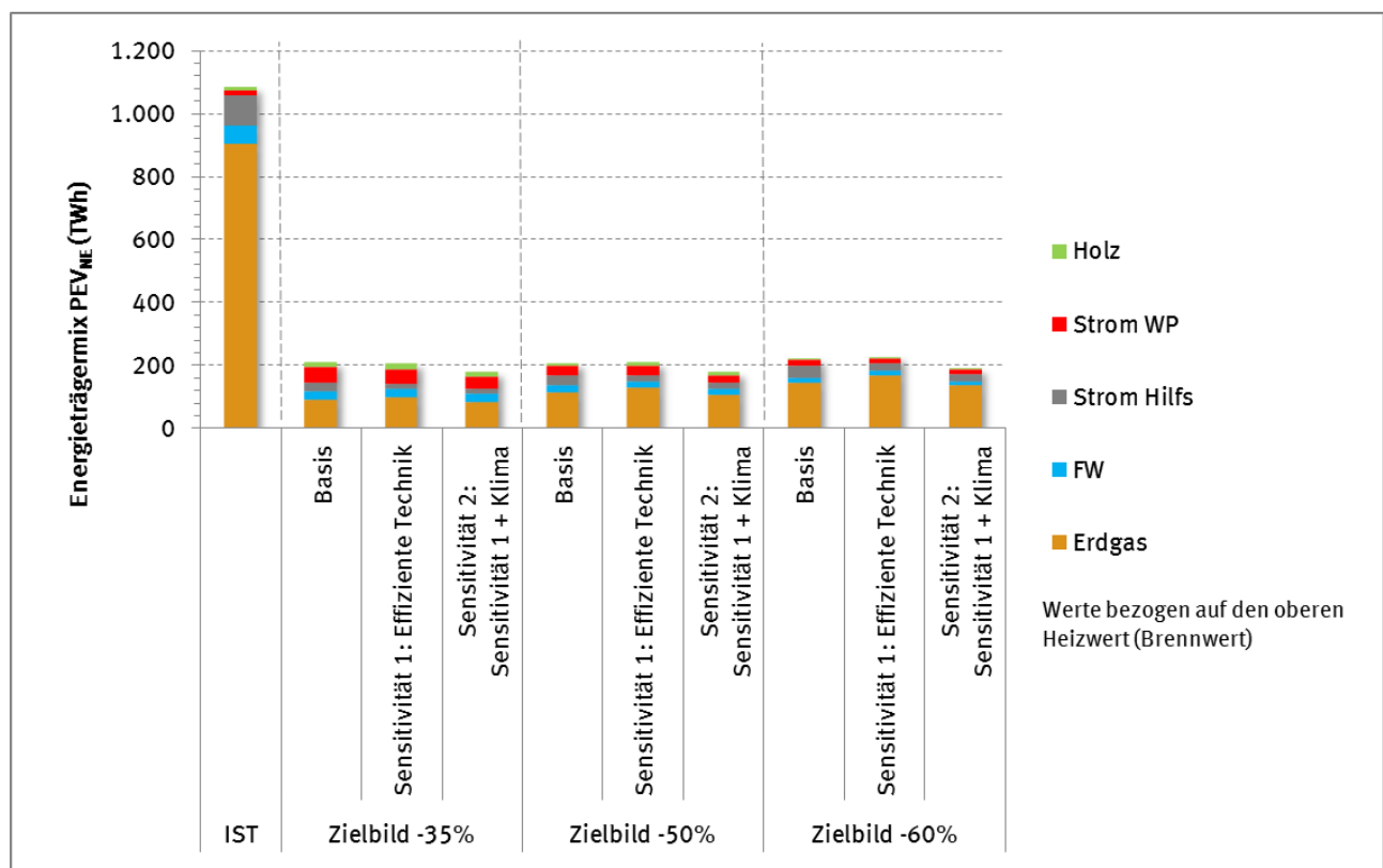
Abbildung 73: Energieträgermix des Verbrauchs nicht-erneuerbarer Primärenergie in den verschiedenen Zielbildern und Sensitivitäten des gesamten Gebäudebestandes
