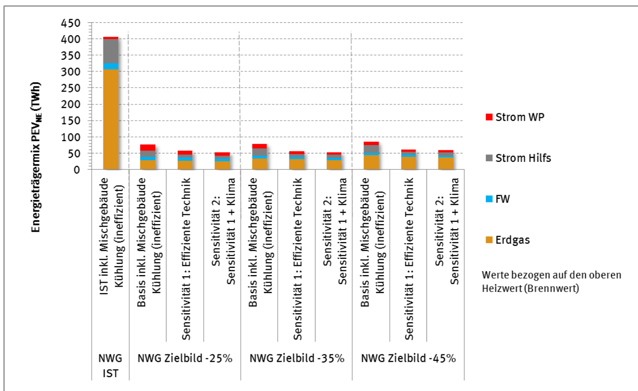
Abbildung 71: Energieträgermix des Verbrauchs nicht-erneuerbarer Primärenergie in den verschiedenen Zielbildern und Sensitivitäten der Nichtwohngebäude
