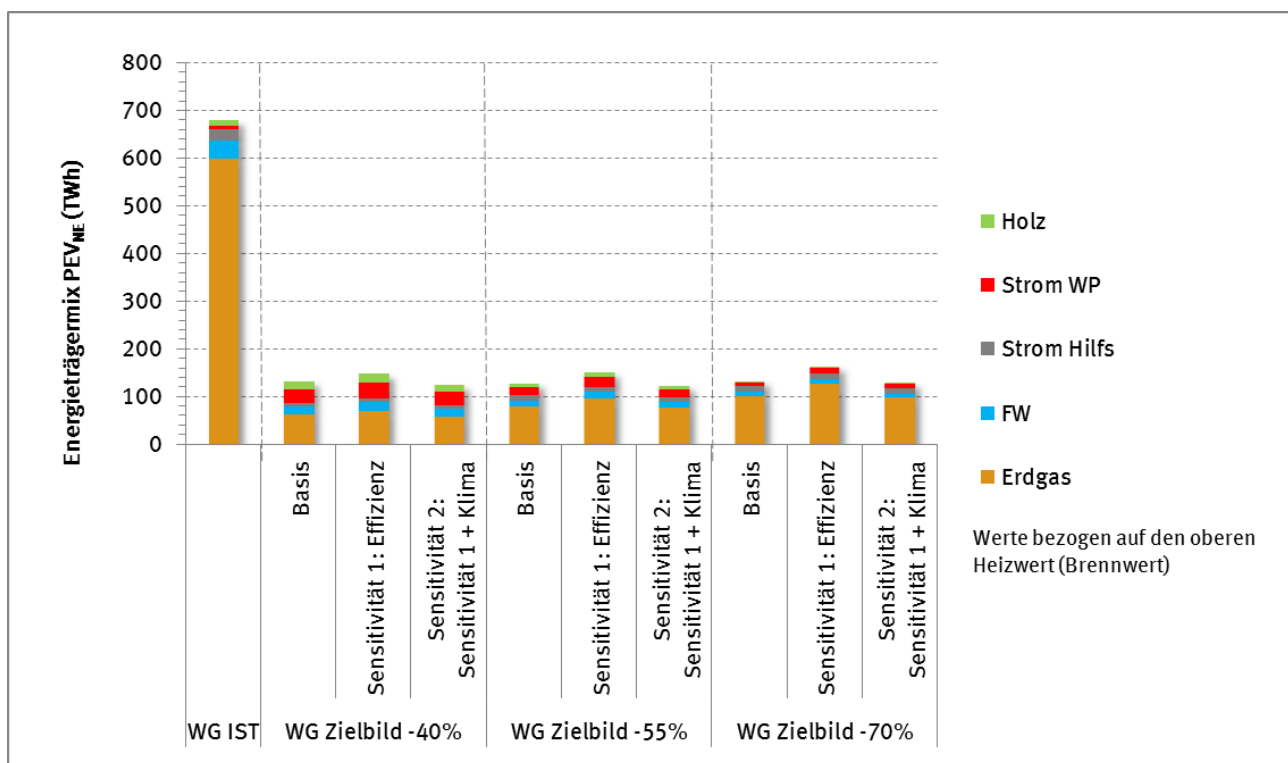
Abbildung 68: Energieträgermix des Verbrauchs nicht-erneuerbarer Primärenergie in den verschiedenen Zielbildern und Sensitivitäten der Wohngebäude
