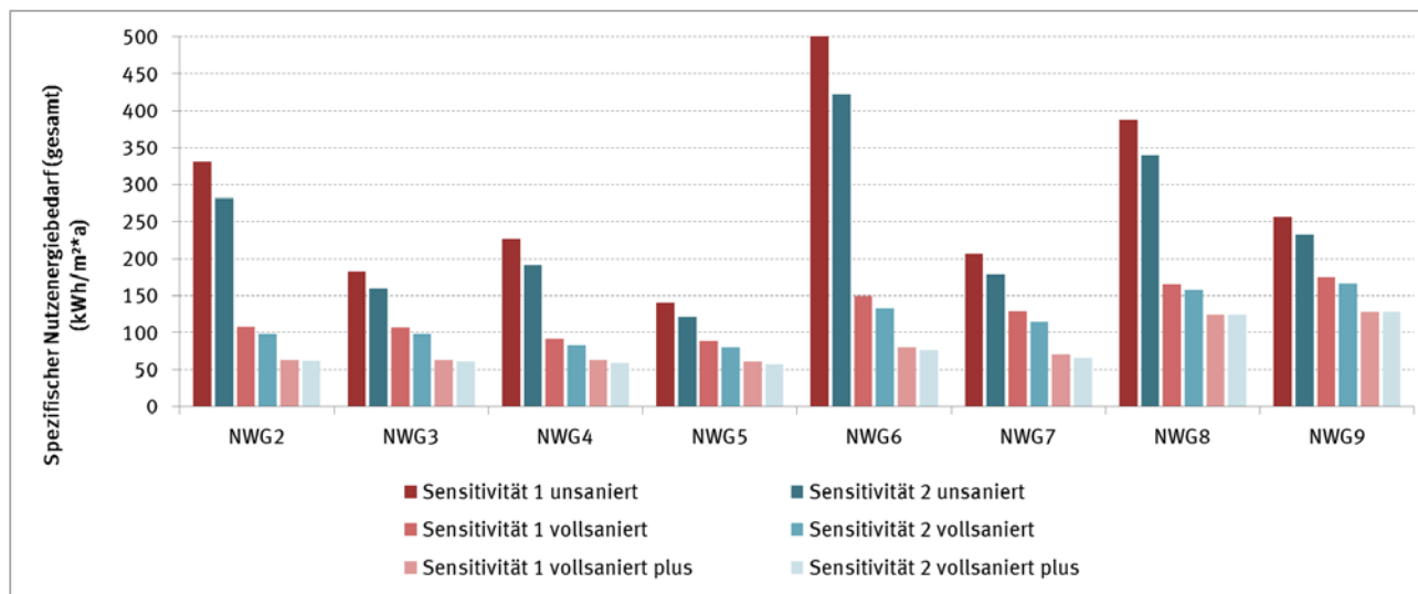
Abbildung 58: Spezifischer Nutzenergiebedarf (gesamt) in vorwiegend durch TABS gekühlten Nichtwohngebäuden (NWG2-9) aufgrund der erwarteten Klimaveränderungen (Referenzstandort Potsdam)
