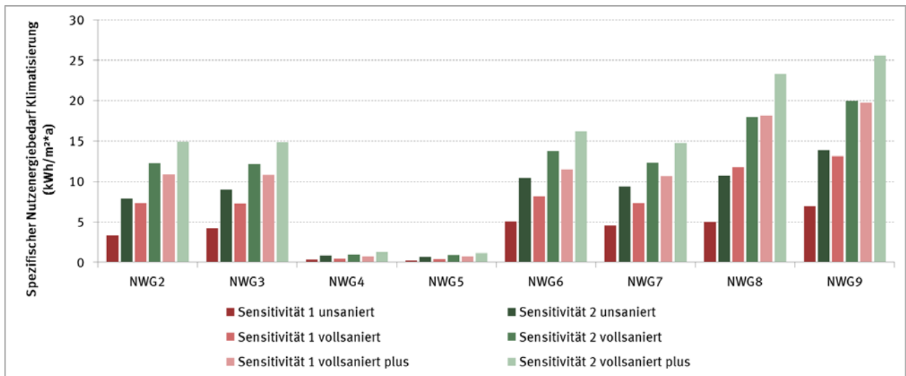
Abbildung 61: Spezifischer Nutzkältebedarf in vorwiegend durch TABS gekühlten Nichtwohngebäuden aufgrund der erwarteten Klimaveränderungen (Referenzstandort Potsdam)
