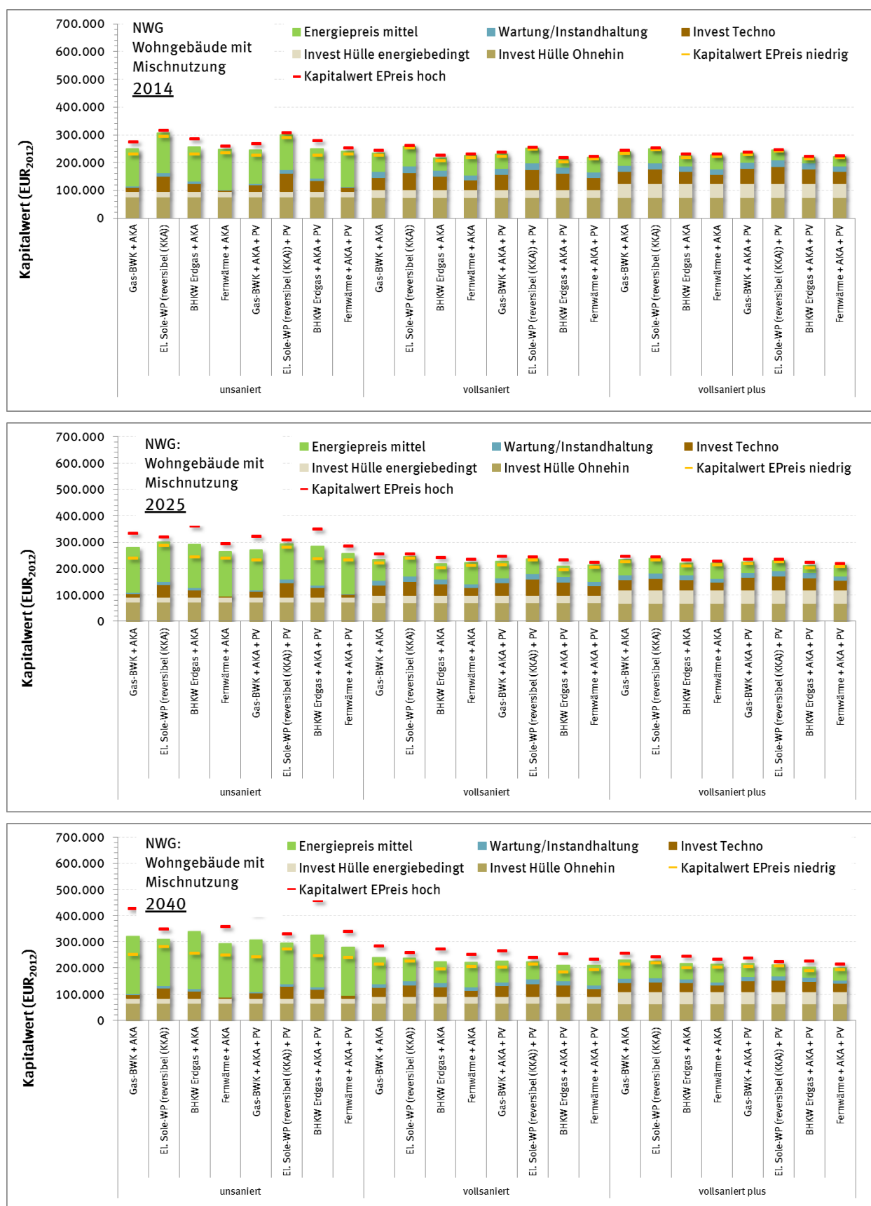
Abbildung 19: Kapitalwerte für ein Nichtwohngebäude mit Mischnutzung in Abh. von Versorgungstechnik, Wärmeschutzstandard und Investitionszeitpunkt
