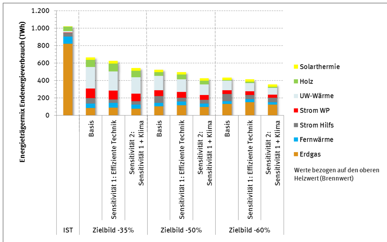
Abbildung 72: Energieträgermix des Endenergieverbrauchs (im Sinne der Energiebilanz) in den verschiedenen Zielbildern und Sensitivitäten des gesamten Gebäudebestandes
