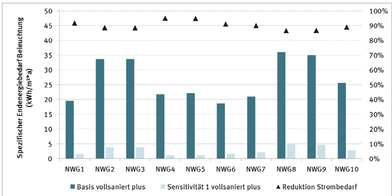
Abbildung 54: Spezifischer Endenergiebedarf für die Beleuchtung in den betrachteten Nichtwohngebäuden im Sanierungszustand „vollsanziert plus“ sowie relatives Einsparpotenzial durch den Einsatz hocheffizienter Beleuchtungsanlagen und einer optimalen Beleuchtungssteuerung
