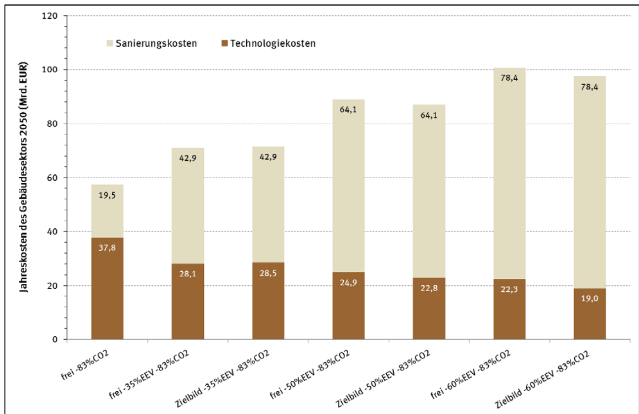
Abbildung 48: Jährliche Kosten des Gebäudesektors bezogen auf das Jahr 2050 unterteilt nach Sanierungskosten (nur energiebedingte Mehrkosten) und Technikkosten in den verschiedenen Szenarien
