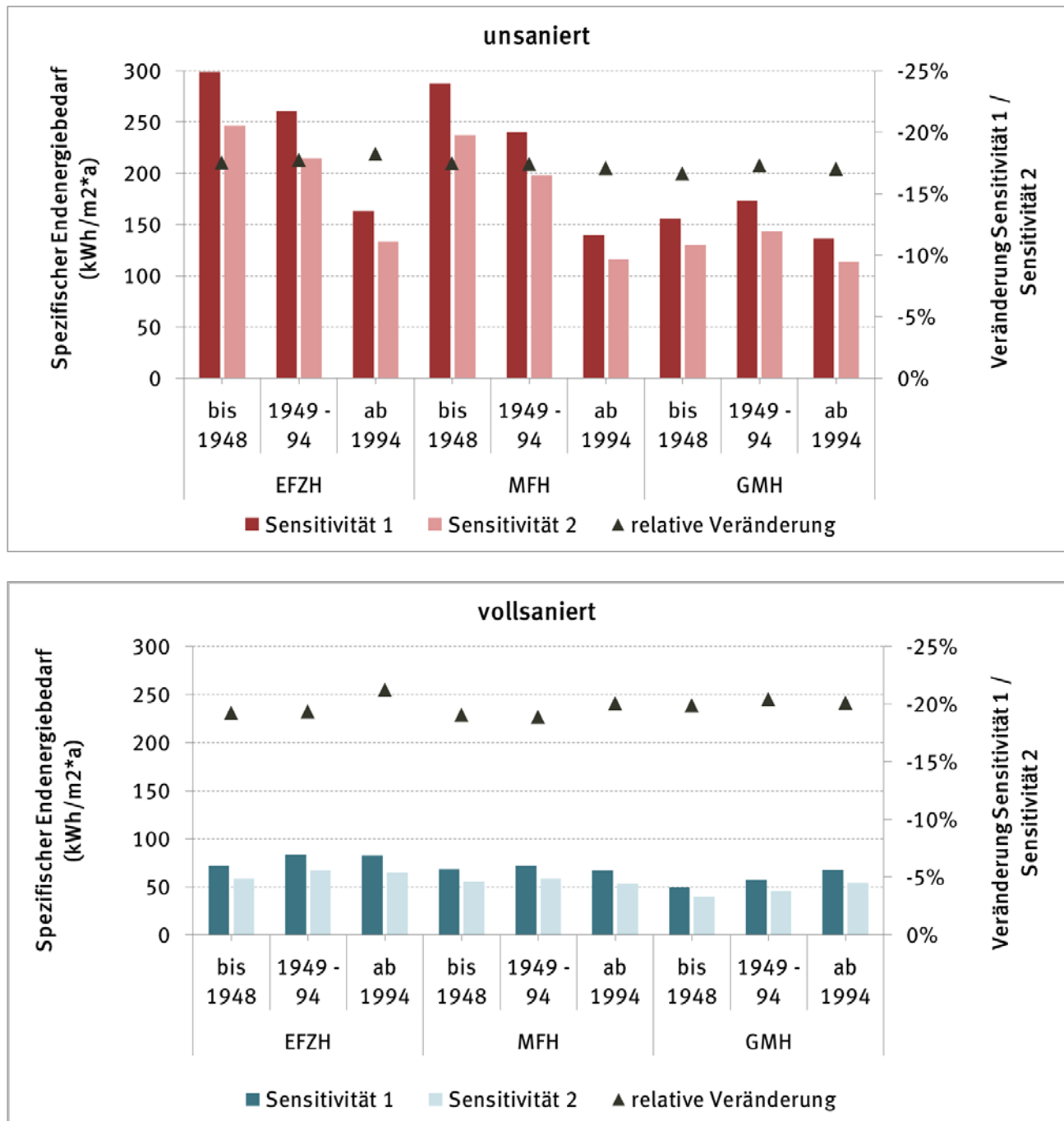
Abbildung 56: Spezifischer Endenergiebedarf für Heizung und TWW in Wohngebäuden (Gas-Brennwert) sowie Veränderungen gegenüber Sensitivität 1 in Abhängigkeit vom Sanierungsstandard
