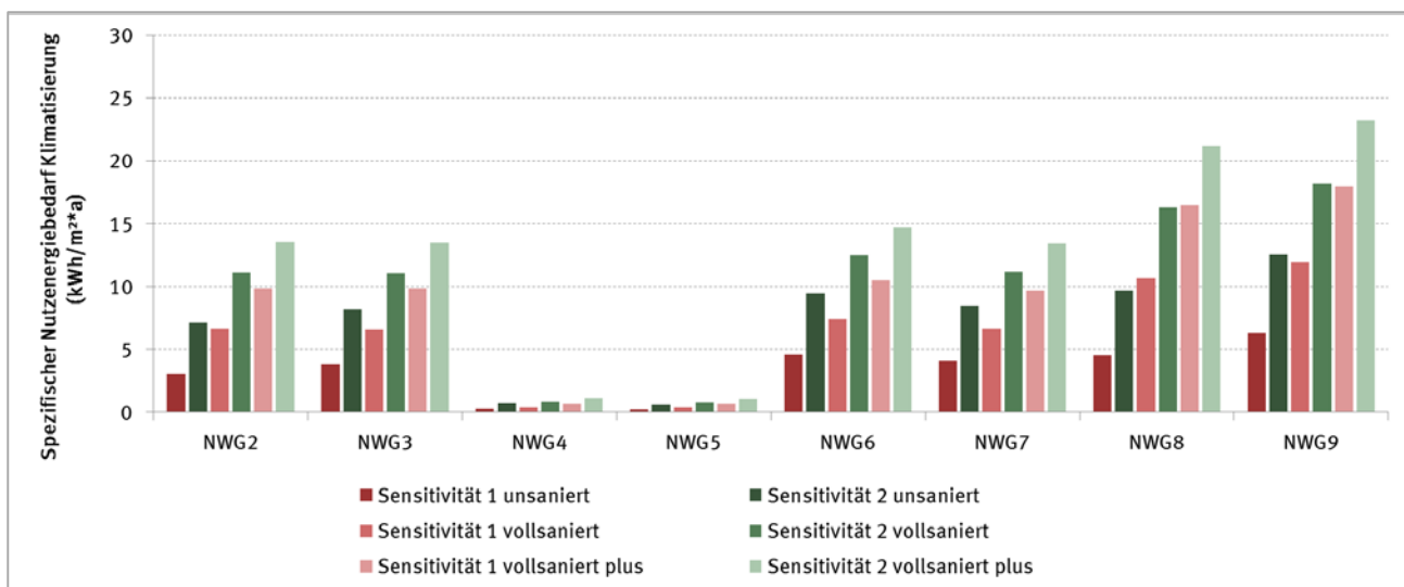
Abbildung 60: Spezifischer Nutzkältebedarf in vorwiegend durch Kühldecken gekühlten Nichtwohngebäuden aufgrund der erwarteten Klimaveränderungen (Referenzstandort Potsdam)
