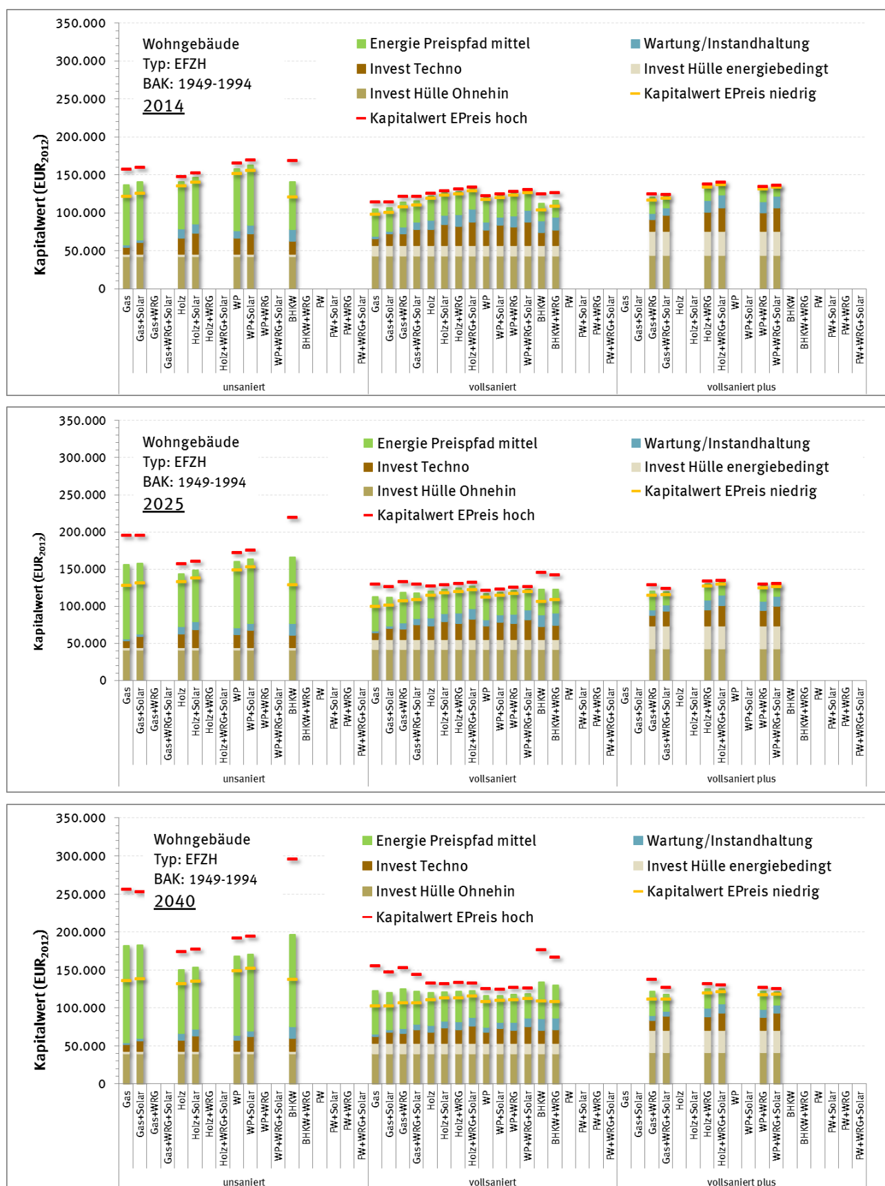
Abbildung 16: Kapitalwerte für ein EFZH in Abh. von Versorgungstechnik, Wärmeschutzstandard und Investitionszeitpunkt
