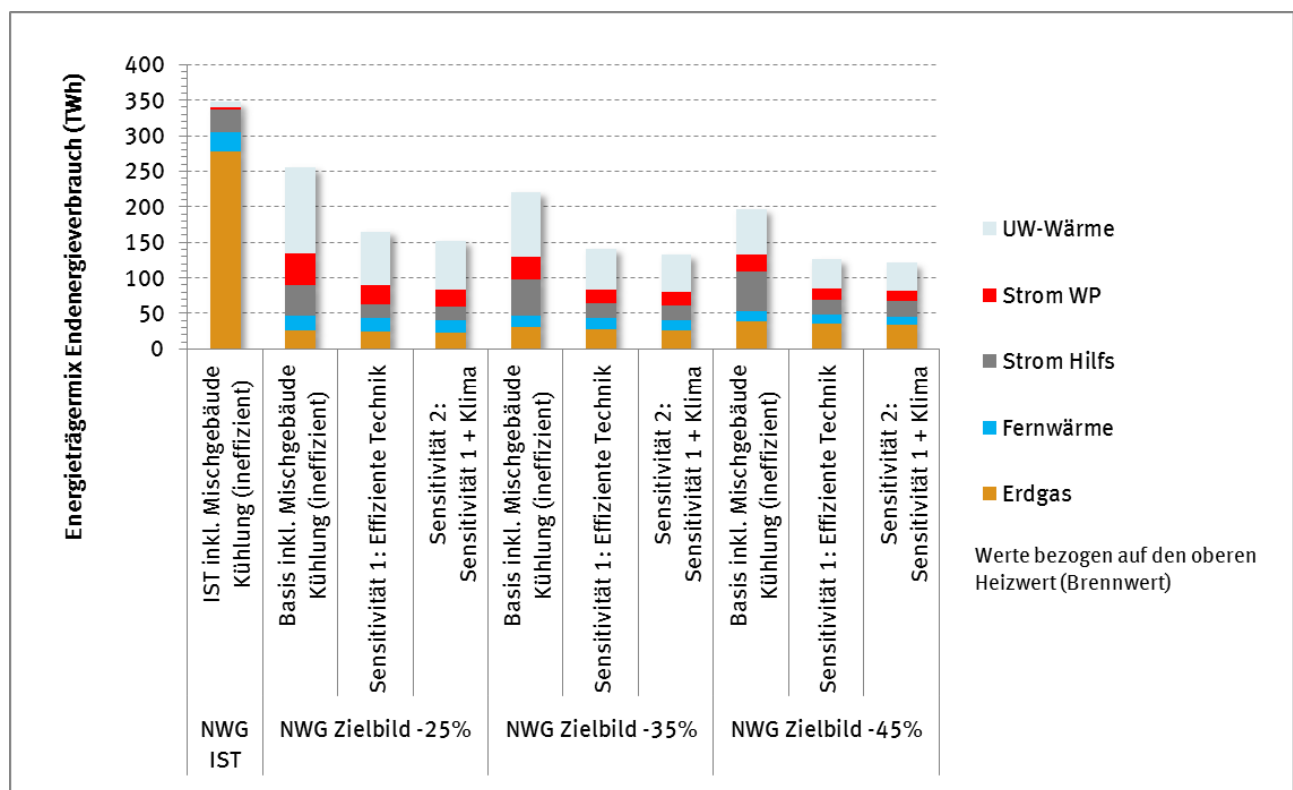
Abbildung 70: Energieträgermix des Endenergieverbrauchs (im Sinne der Energiebilanz) in den verschiedenen Zielbildern und Sensitivitäten der Nichtwohngebäude
