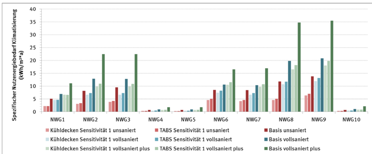
Abbildung 52: Spezifischer Kältenutzenergiebedarf der betrachteten Nichtwohngebäude in Abhängigkeit von Sanierungsstandard und überwiegendem Kälteübertragungssystem
