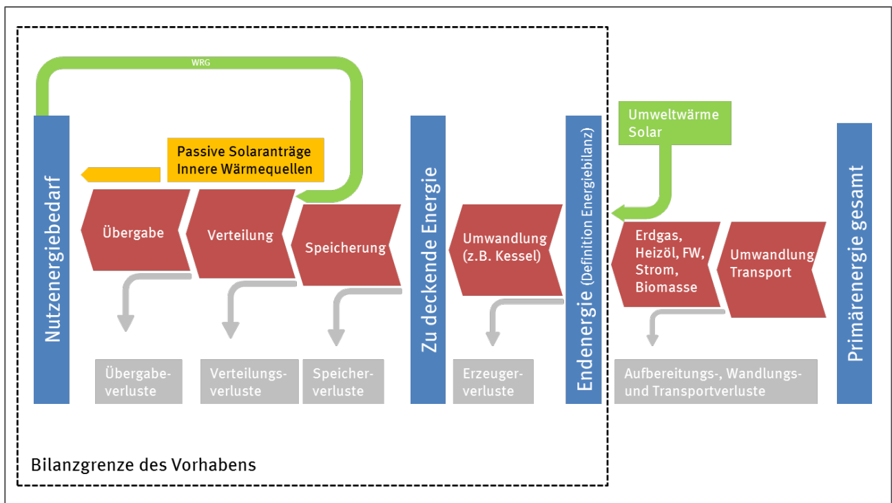
Abbildung 3: Schematisches Energieflussbild
