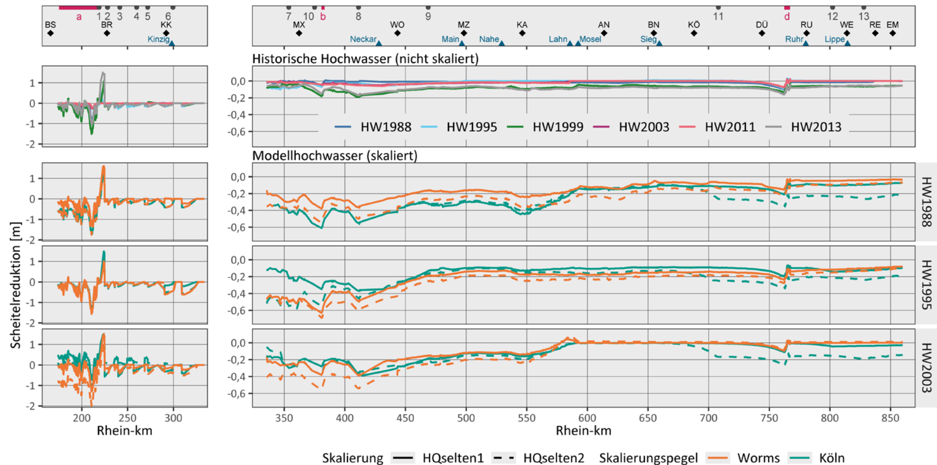
Abbildung 8: Längsschnitte der Wasserspiegeldifferenzen am Rhein zwischen Bezugzustand und Planzustand 2027+ (alle Maßnahmen im Flussgebiet) für die 18 im FuE-NHWSP modellierten Hochwasser
