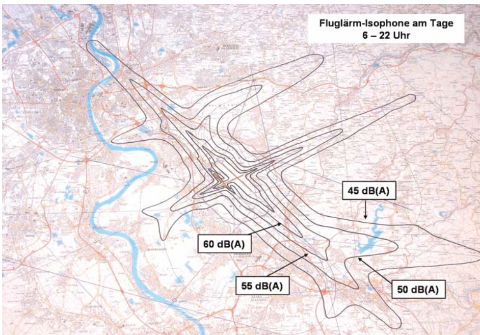
Abbildung 1. Isophone für Fluglärm am Tage (6 – 22 Uhr)
