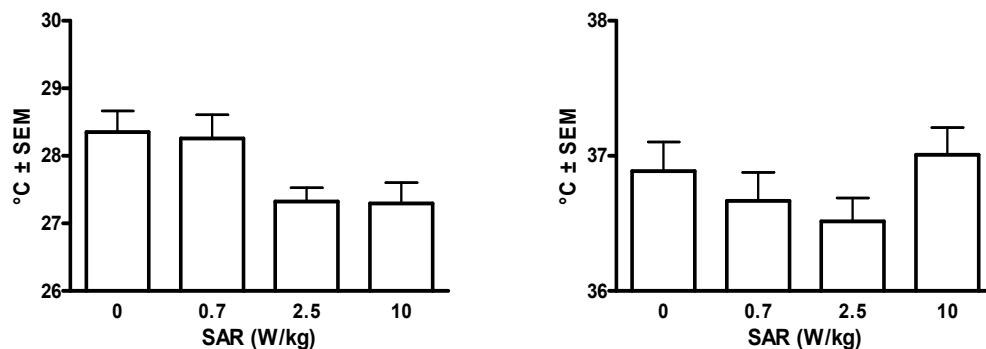
Abb. 12: Hautoberflächentemperaturen (a) und Körperkerntemperaturen (b) exponierten bzw. scheinexponierten Ratten (Mittelwerte ± SEM).
